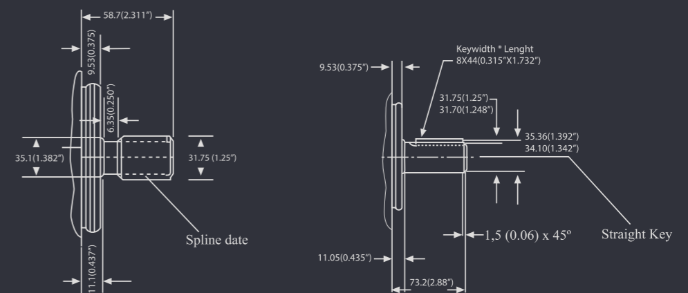
شافت هزارخار (14spl)
